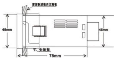
面板(嵌入)式安装 开孔尺寸为: 45X45mm
