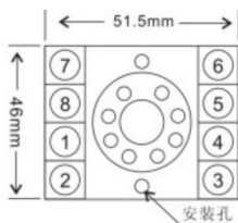
基座(导轨)安装座 置入35mm导轨中
