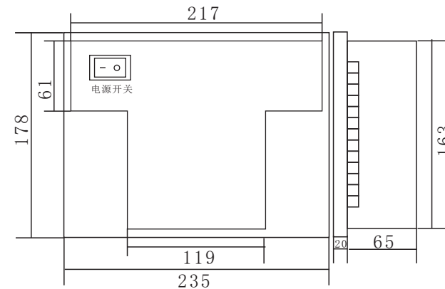
外形尺寸: 235×178×85
